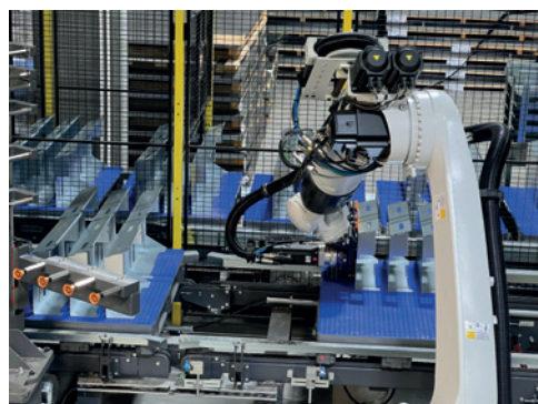
Die LVD Biegezone Ulti-Form biegt Teile bis zu einer Größe von 1200 mal 800 mm vollautomatisch und mannlos.
