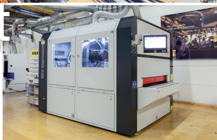
Schleifzentrum Impression mit Tellerschleif- und Bürstaggregat von Heesemann
